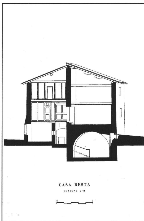
Fig. 11 - Sezione trasversale
