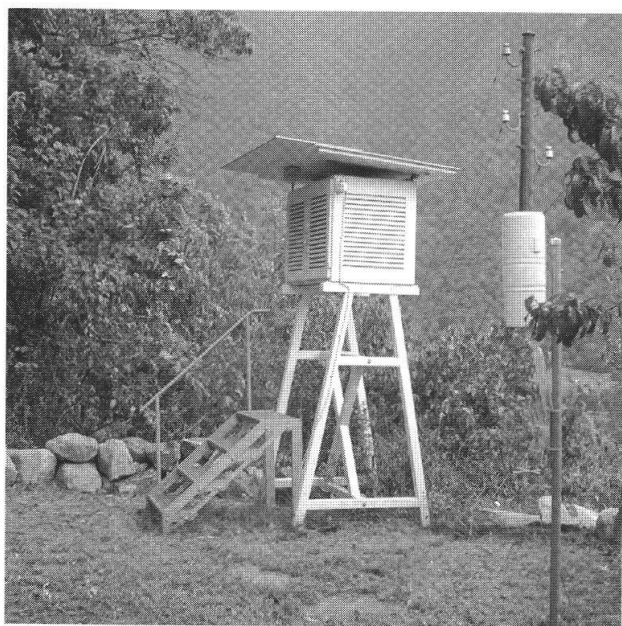
Capannina meteorologica e pluviometro della stazione di Grono.
