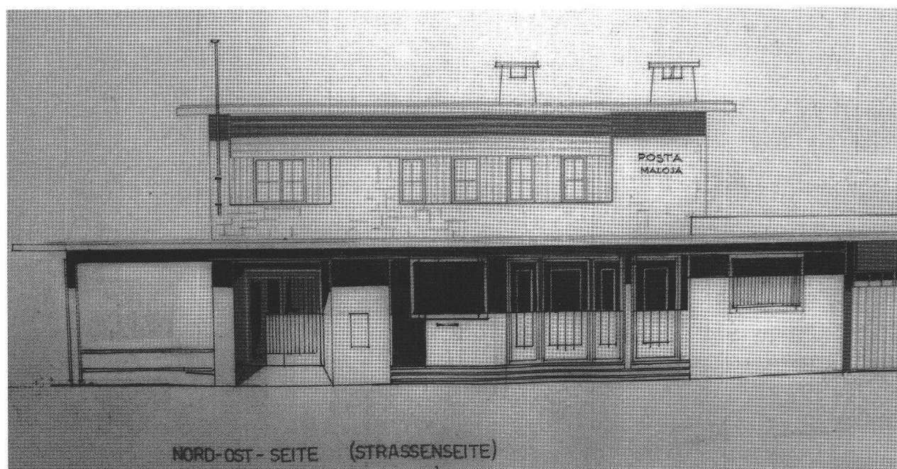
Maloja/Maloggia, posta, prospetto della facciata principale. Archivio di Stato dei Grigioni.
