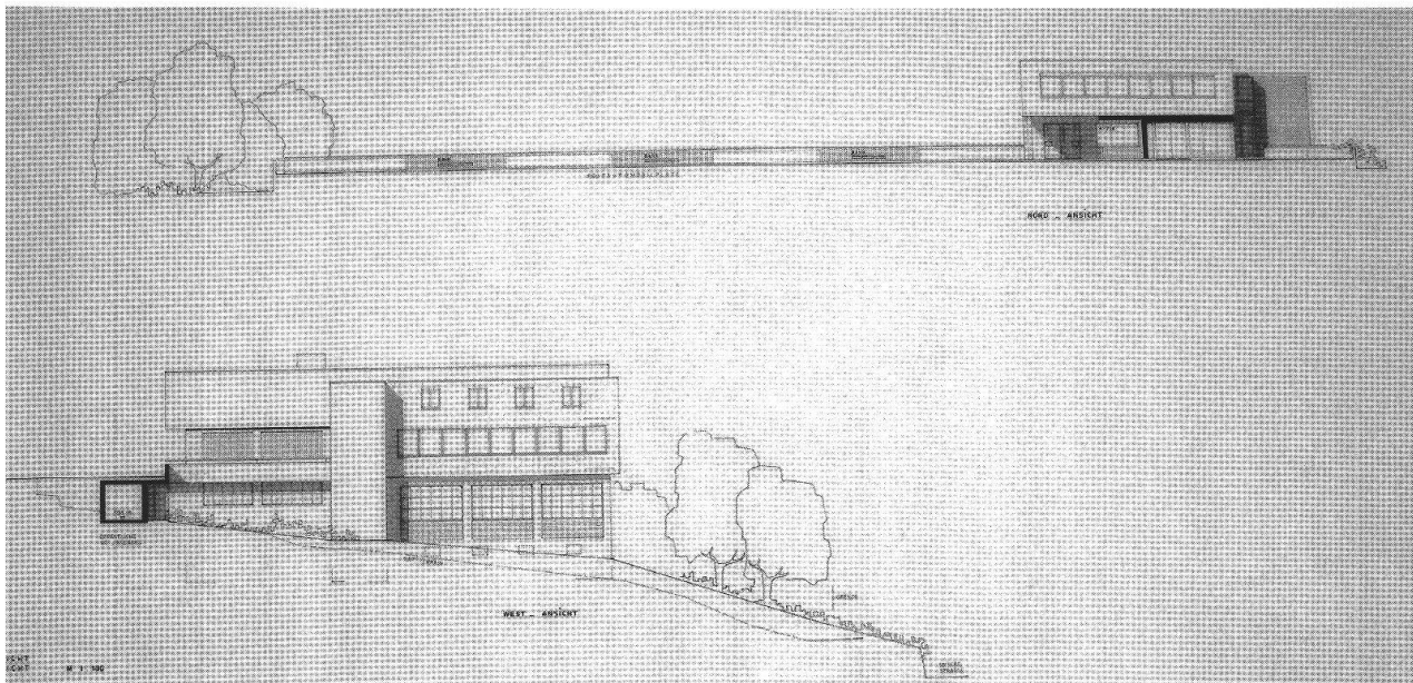
Scuol, posta, prospetti delle facciate nord e ovest. Archivio di Stato dei Grigioni.
