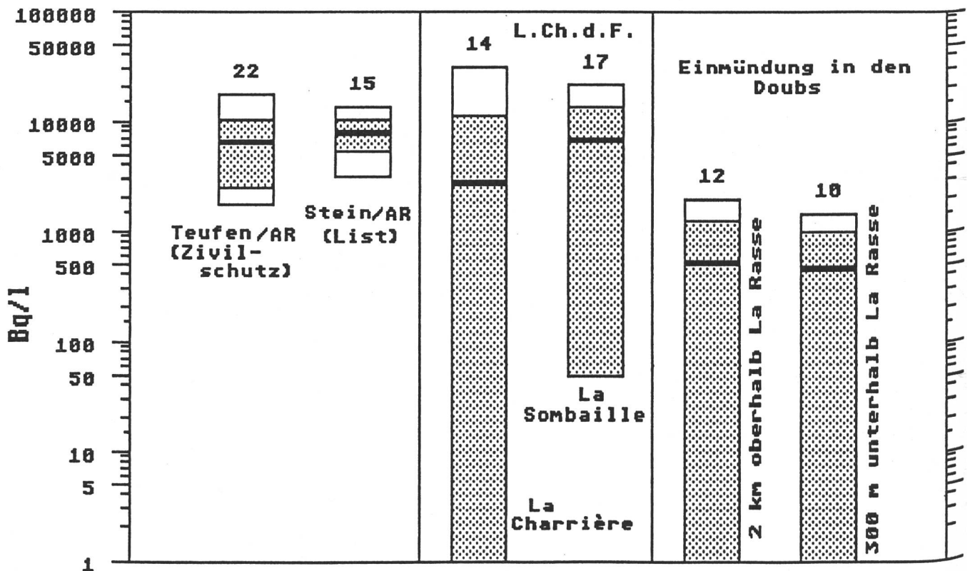
Fig.4.1.b: Tritium in Sickerwasser aus Deponien (1982-86)
