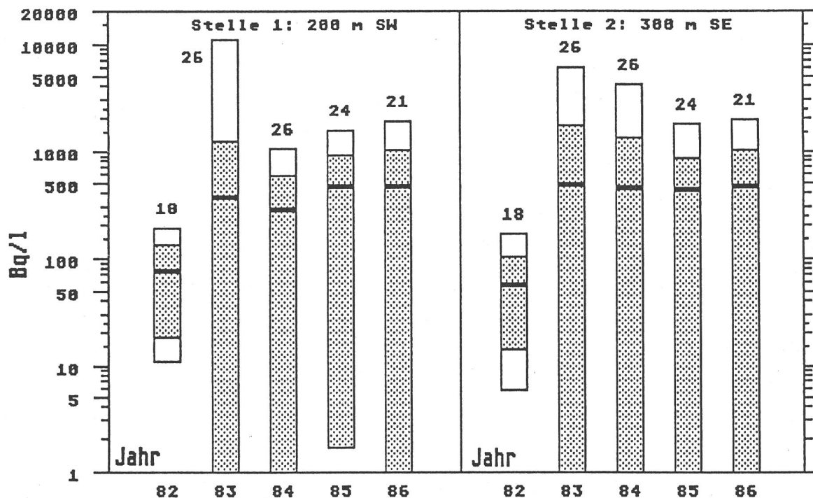
Fig.4.2.b: Tritium im Niederschlag Umgebung MB Microtec, Niederwangen/BE
