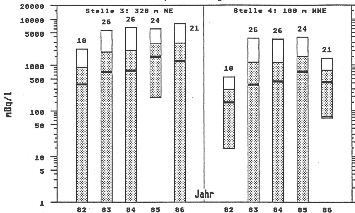
Fig.4.2.c: Tritium im Niederschlag Umgebung MB Microtec, Niederwangen/BE
