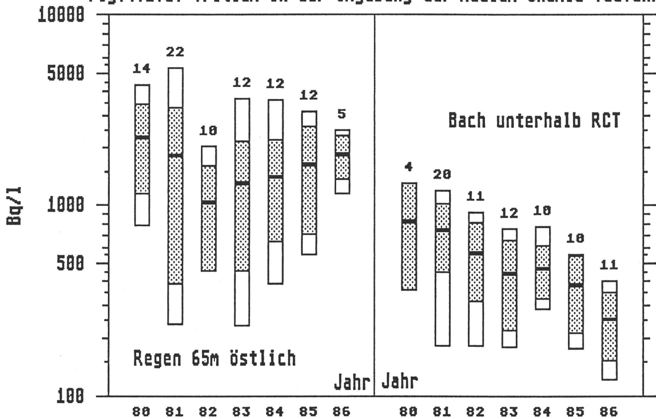
Fig.4.1.a: Tritium in der Umgebung der Radium-Chemie Teufen/AR
