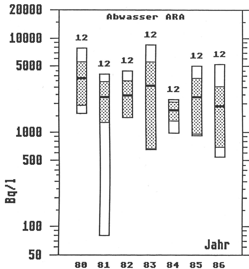
Fig.4.3 (a,b): Tritium in der Gegend von La Chaux-de-Fonds
