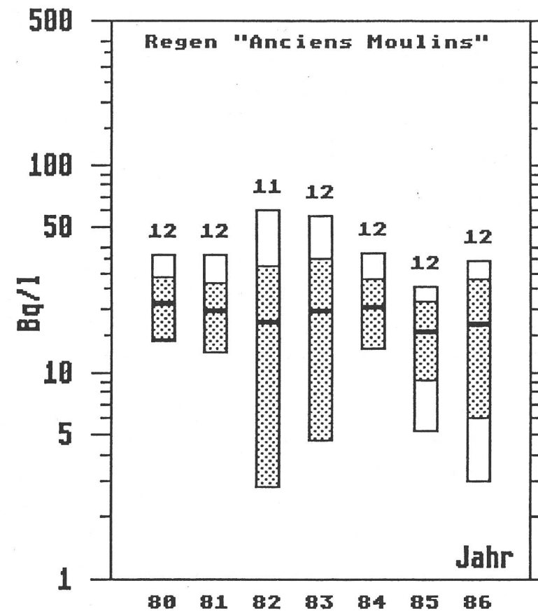
Fig.4.3 (a,b): Tritium in der Gegend von La Chaux-de-Fonds
