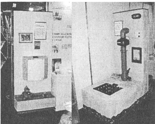
Figur 17: Sanierungsmodelle im Massstab 1:1
