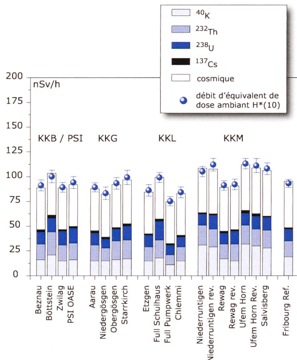
Figure 1: Contributions individuelles au débit d'équivalent de dose ambiant H*(10) calculées à partir des spectres in situ (distribution supposée homogène des radionucléides dans le sol) mesurés au voisinage des centrales nucléaires suisses en 2009. La mesure globale du débit d'équivalent de dose ambiant H*(10) avec chambre d'ionisation est également représentée.
