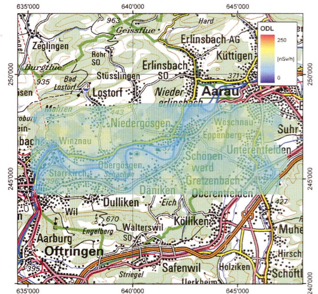
Figur 3: Karte der Ortsdosisleistung im Messgebiet KKG. Kartendaten PK200 © swisstopo (DV084391).
