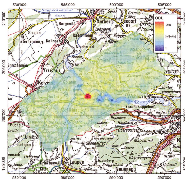
Figur 2: Karte der Ortsdosisleistung im Messgebiet KKM. Kartendaten PK200 © swisstopo (DV084391).
