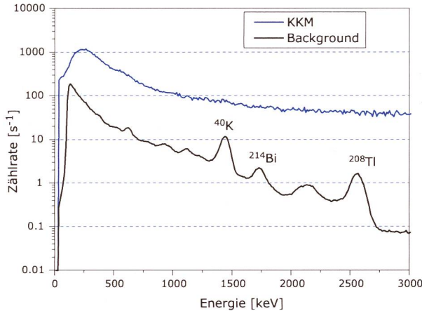
Figur 1: Photonenspektrum über dem KKM im Vergleich zum Untergrund. Das KKM-Spektrum wird dominiert durch die gestreute, hochenergetische Photonenstrahlung des ^{16}\text{N} (Photopeak bei 6.1 MeV). Beim Untergrundspektrum können die Photonenmissionen der natürlichen Radionuklide ^{40}\text{K} , ^{214}\text{Bi} und ^{208}\text{Tl} erkannt werden.
