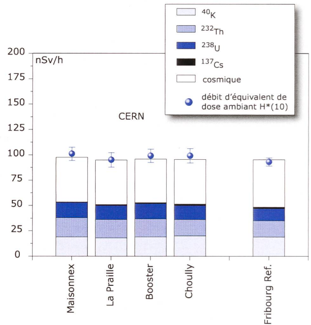
Figure 2: Contributions individuelles au débit d'équivalent de dose ambiant H*(10) calculées à partir des spectres in situ (distribution supposée homogène des radionucléides dans le sol) mesurés en 2009 au voisinage du CERN ainsi qu'au point de référence de Fribourg. La mesure globale du débit d'équivalent de dose ambiant H*(10) avec chambre d'ionisation est également représentée.
