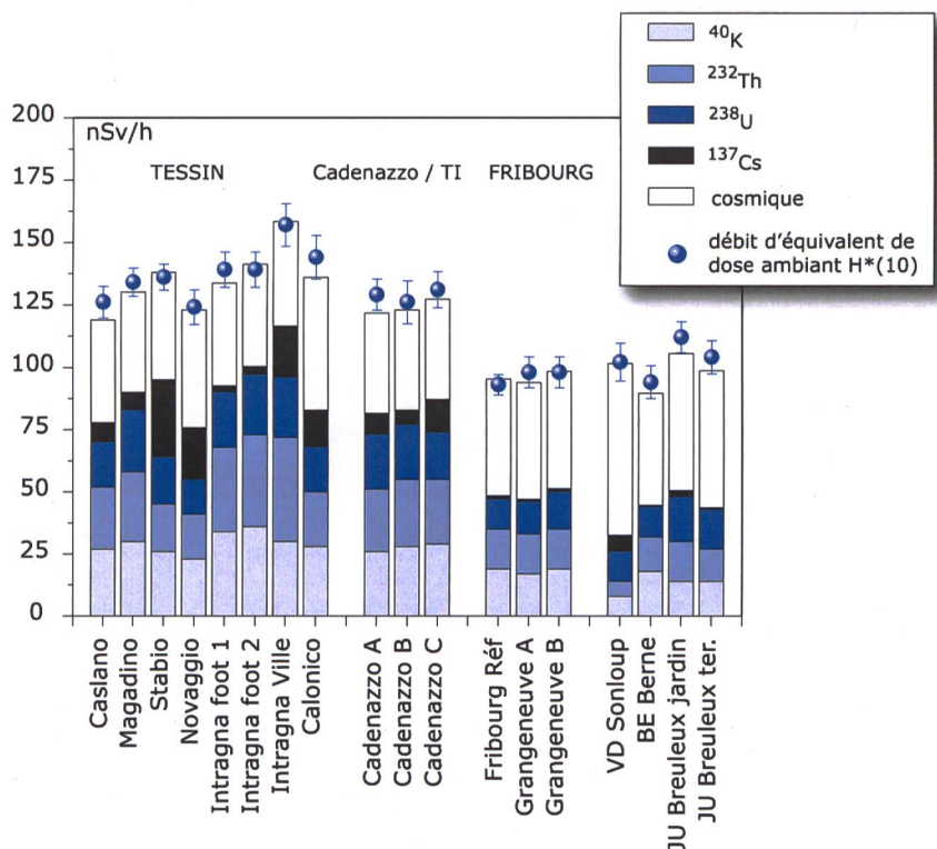
Figure 3: Contributions individuelles au débit d'équivalent de dose ambiant H*(10) calculées à partir des spectres in situ (distribution supposée homogène des radionucléides dans le sol) mesurés en 2009 au Tessin ainsi que dans le canton de Fribourg. La mesure globale du débit d'équivalent de dose ambiant H*(10) avec chambre d'ionisation est également représentée.
