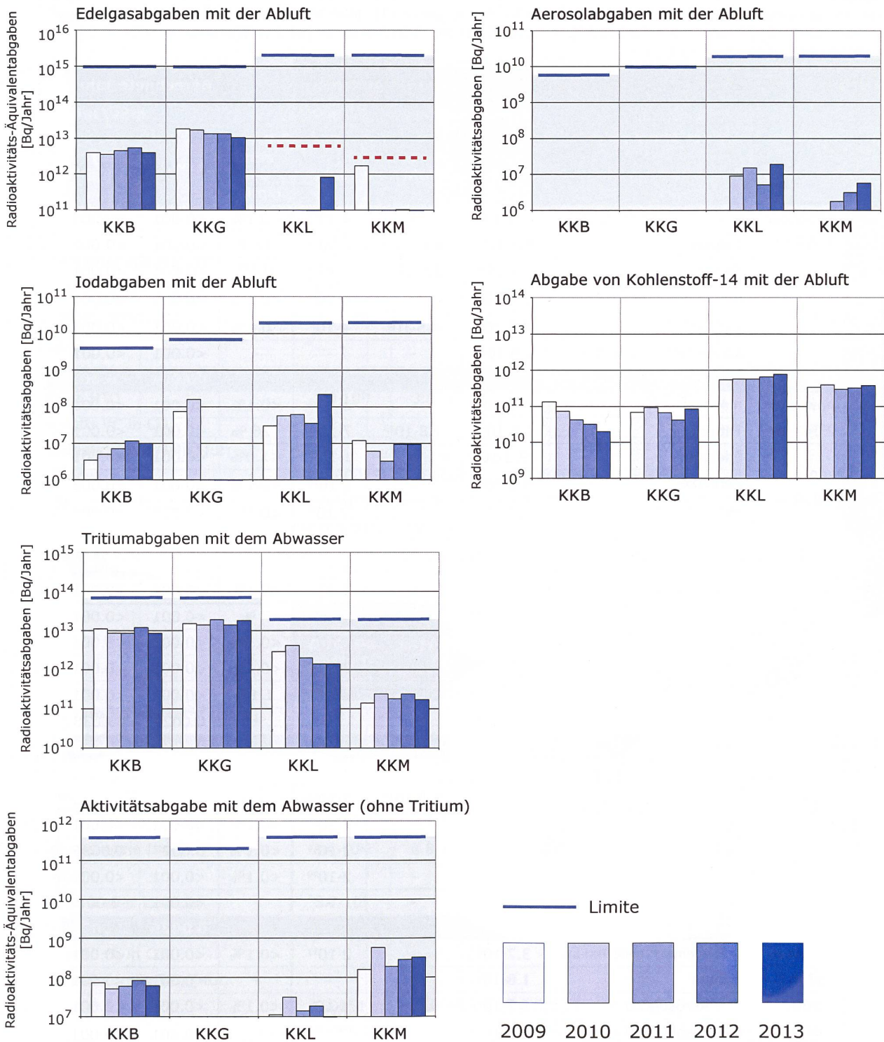
Figur 1: Abgaben der schweizerischen Kernkraftwerke an die Atmosphäre in den letzten fünf Jahren (2009 bis 2013) im Vergleich mit den Jahres-Abgabelimiten.
