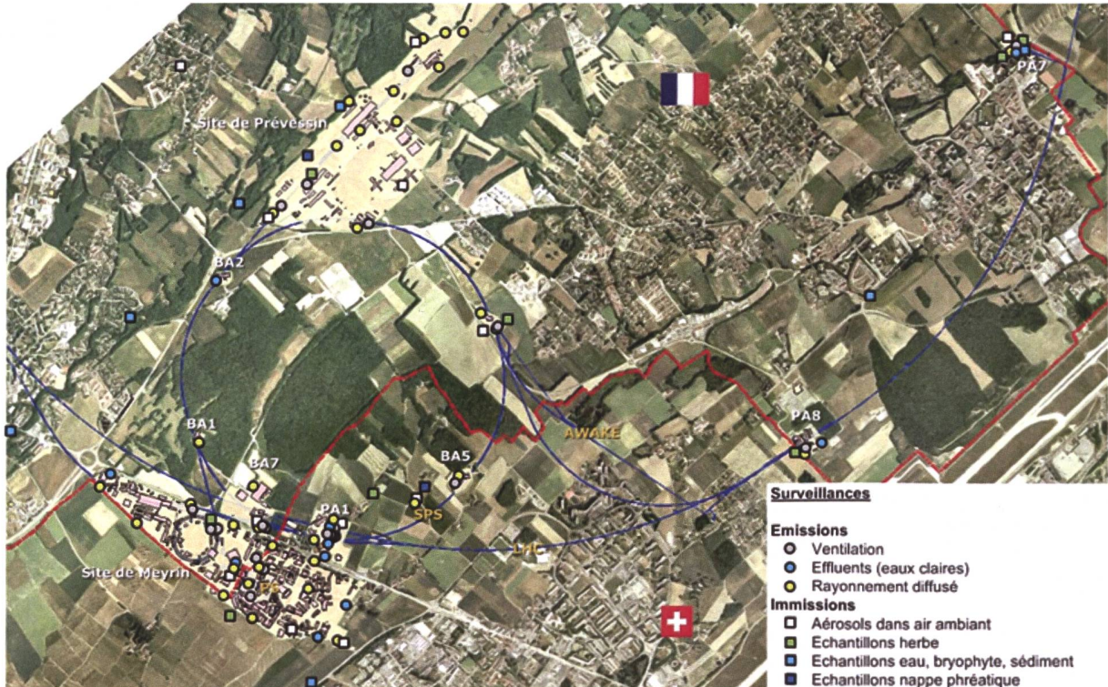
Figure 2: Région frontalière franco-suisse: sites de Meyrin et de Prévessin du CERN, implantation de l'anneau du Super synchrotron à proton (SPS) et du Grand collisionneur d'hadrons (LHC), situation des stations de surveillance et lieux d'échantillonnage du CERN; ceux qui concernent le territoire suisse y sont tous représentés, excepté le point de collecte des échantillons de l'Allondon qui est hors-carte.
