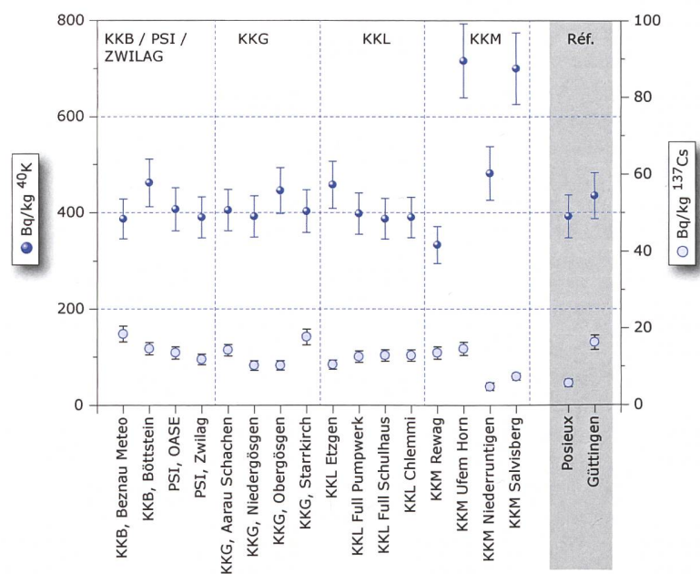
Figure 3: ^{137}\text{Cs} et ^{40}\text{K} (naturel) dans les sols secs et tamisés (2 mm) analysés par l'OFSP en 2013 (couche 0 - 5 cm). Les valeurs mesurées à Posieux et Güttingen sont représentées à titre de comparaison (grisées).
