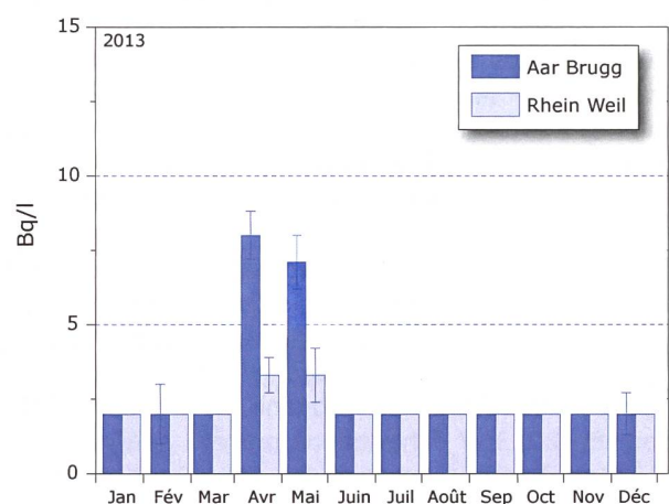
Figure 4: Suivi du tritium dans les échantillons mensuels d'eau de l'Aar à Brugg/AG et du Rhin prélevés à Weil/D en 2013.
