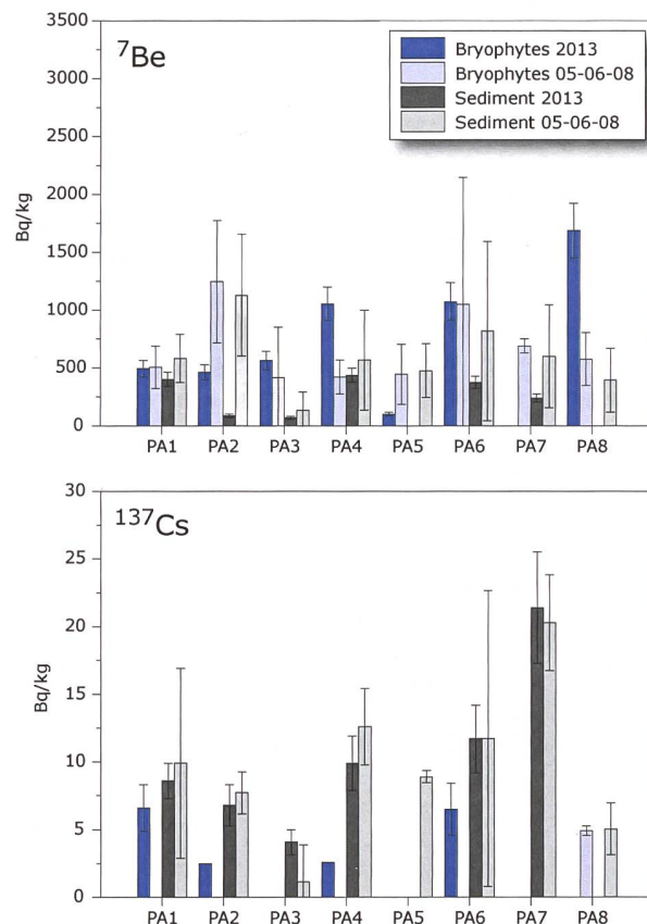
Figure 4 : Activités du ^7\text{Be} et du ^{137}\text{Cs} dans les bryophytes et les sédiments aux points de rejet du LHC en 2013. Les valeurs 05-06-08 correspondent aux moyennes des résultats des campagnes de mesures effectuées au cours des périodes témoins 2005-2006-2008.
