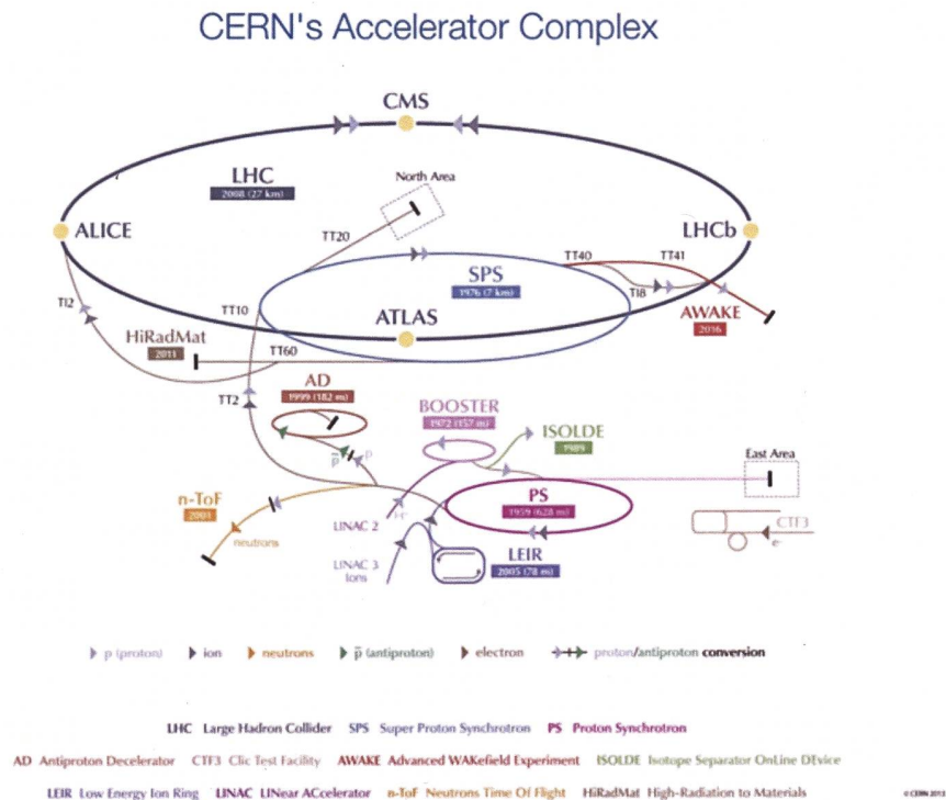
Figure 1: La complexe des accélérateurs du CERN (voir Glossaire en fin de chapitre).
