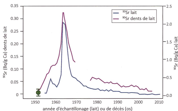
Figure 1 : Activités en ^{90}\text{Sr} dans le lait (en bleu) et dans les dents de lait (en rouge) mesurées en Suisse de 1951 à 2016. Le point en vert indique la mesure de contrôle effectuée en 2016 sur un échantillon de dents de lait provenant d'un individu né en 1951. L'absence de données entre 1970 et 1975 provient de l'interruption du programme de mesure, repris suite à l'accident de Tchernobyl.
