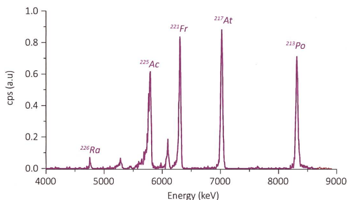
Figure 2 : Spectre alpha de la fraction radium électro-déposée sur disque d'Ag + , à partir de 500 ml d'urine après séparation chimique. On identifie le ^{226}\text{Ra} , ainsi que les filles du traceur ^{225}\text{Ra} , ^{225}\text{Ac} , ^{221}\text{Fr} , ^{217}\text{At} et ^{213}\text{Po} . On utilise le pic de ^{217}\text{At} pour la mesure du traceur, car sa ROI est exempte d'interférence et la probabilité d'émission alpha sur sa ligne est de 100%.
