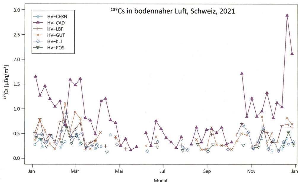
Figur 1: ^{137}\text{Cs} Konzentrationen in der Luft für das Jahr 2021.
