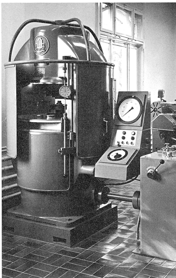
In dieser hydraulischen Senkpresse wird das positive Original auf einen negativen Prägestempel übernommen. (Bilder: zvg)
