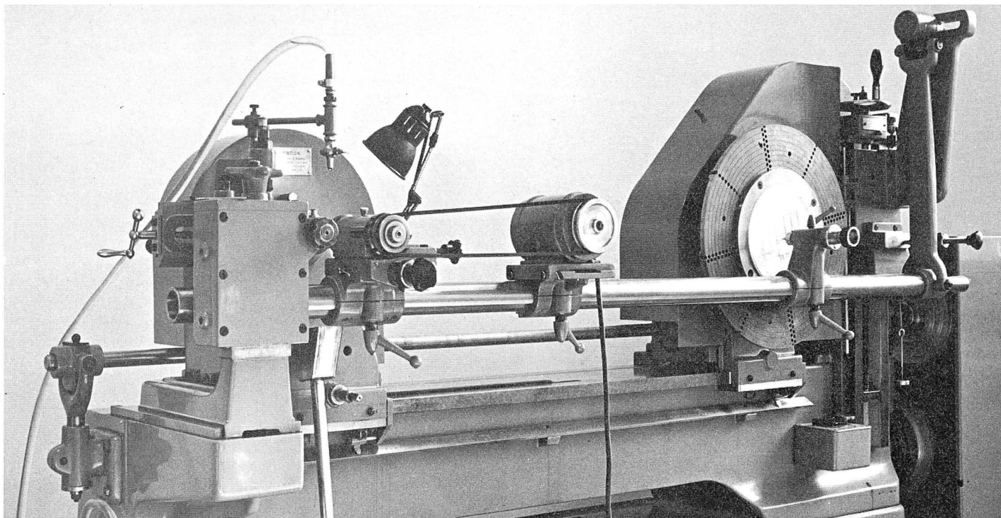
Rechts auf diesem Pantograph ist die grosse Modellmünze zu erkennen. Die Maschine verkleinert und graviert das Sujet nun als posi-
