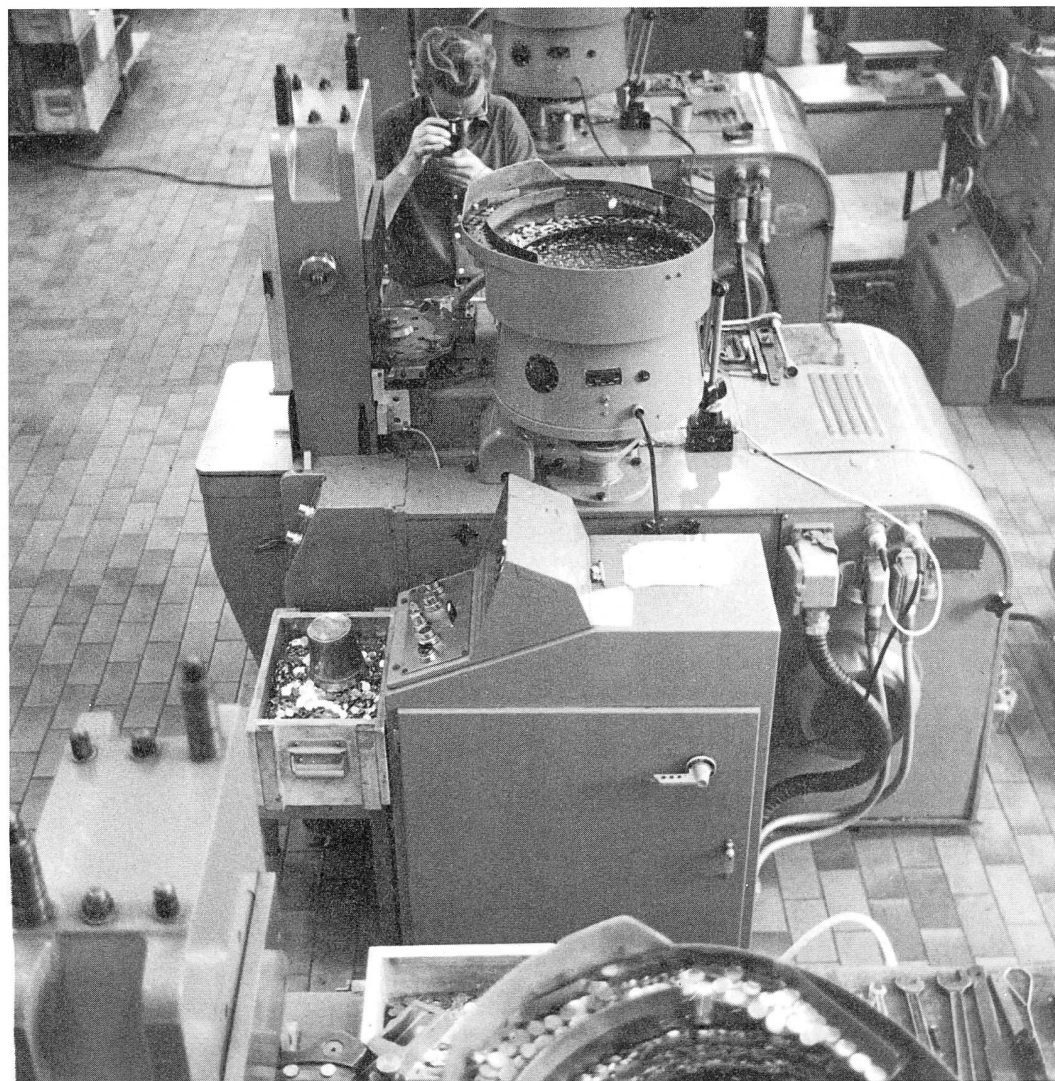
Blick in den Prägesaal der eidgenössischen Münzstätte in Bern; mit den 12 modernen Prägepressen können täglich bis 1,1 Millionen Münzen geprägt werden.
