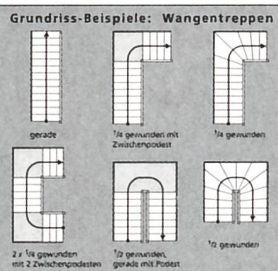
Grundriss-Beispiele: Wangentreppen
