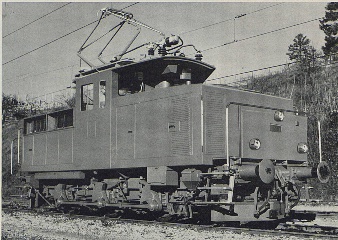
Locomotive de manœuvre de la série Ee 3\frac{1}{3} IV prévue pour quatre systèmes de courant: 15 kV 16\frac{2}{3} Hz (CFF), 3 kV courant continu (FS, Chiasso), 1,5 kV courant continu (SNCF, Genève), 25 kV 50 Hz (SNCF, Bâle)
