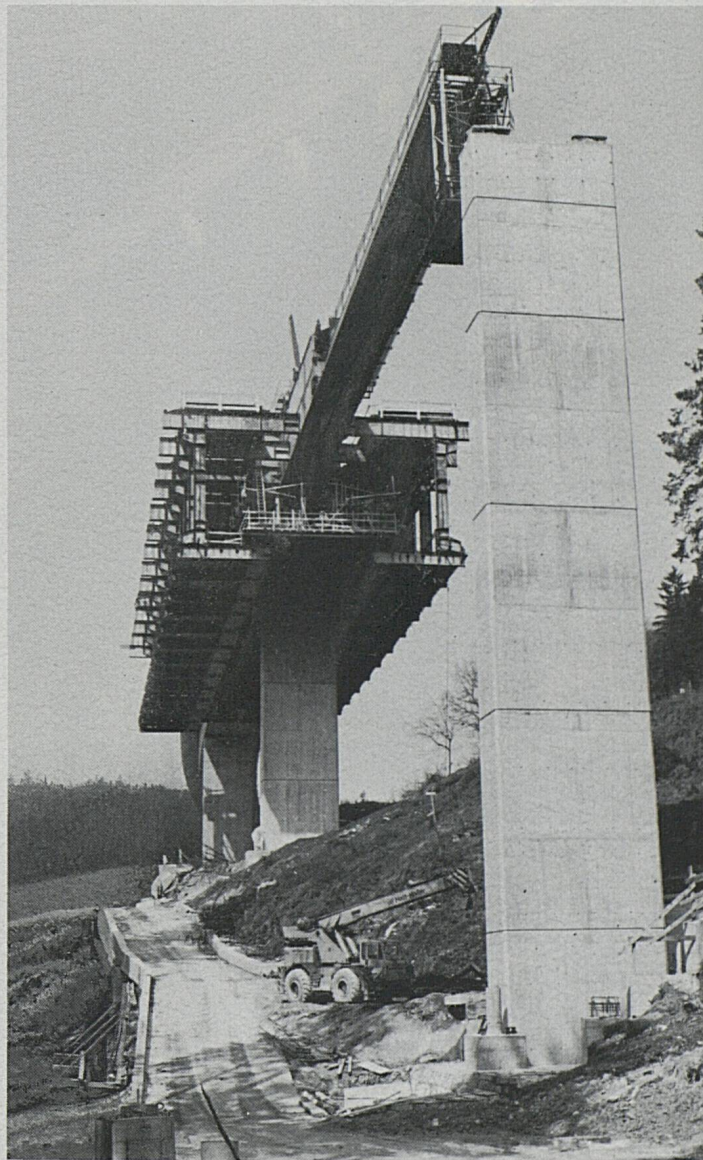
Portique de coffrage avec flèche de lancement
