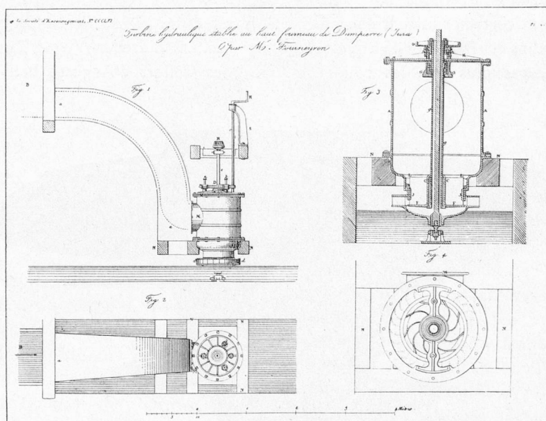
Première turbine commandée à Fourneyron en 1832
