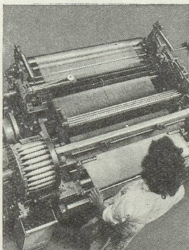
Notre couverture : Métier automatique moderne RUTI, à une navette du modèle BAN à bâti surbaissé
