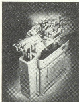
Tour automatique à découper « Tornos » type R-10 avec passage de barre de 11,5 mm. Usines Tornos S. A., Moutier (Suisse). Fondée en 1880.
