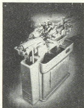
Tour automatique à décoller « Tornos » type R-10 avec pas- sage de barre de 11,5 mm. Usines Tornos S. A., Moutier (Suisse). Fondée en 1880.
