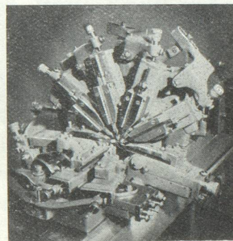
Les 6 outils radiaux d'un tour à décolleter.
