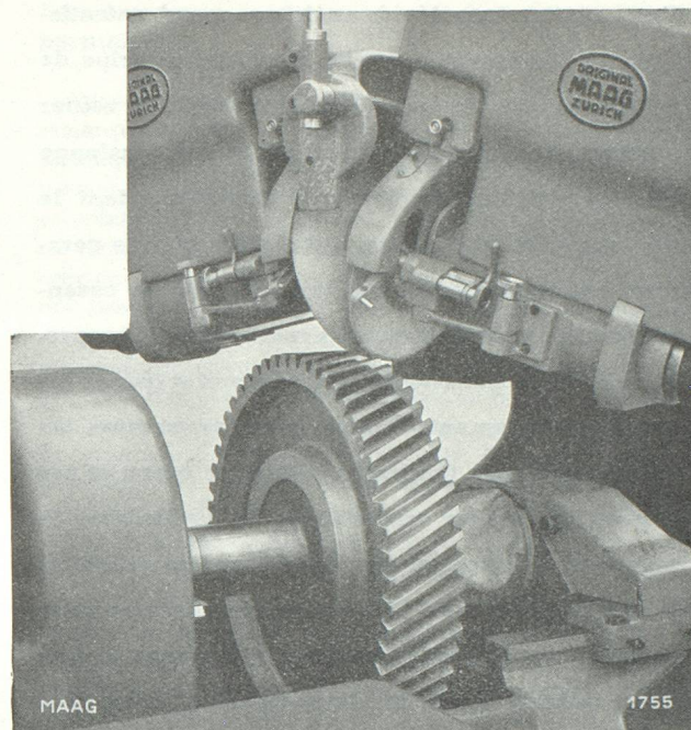
Machine MAAG à rectifier les engrenages droits et hélicoïdaux jusqu'à 300 mm. de diamètre. Rectification selon le procédé de génération.
