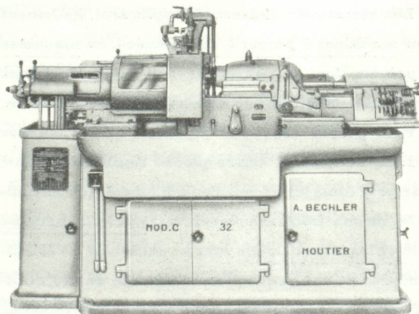
Tour automatique à décolleter à poupée mobile.
