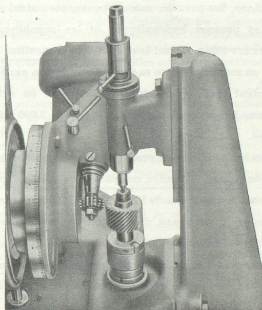
Machine à tailler universelle Mikron type 102. Agent français : A. Moynet SA, Paris-IV e .
