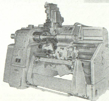
Les 6 outils radiaux d'un tour à décolleter.
