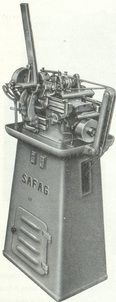
Machine à tailler les engrenages par division, 1-3 fraises, chargeur automatique (SAFAG SA, Bienne).
