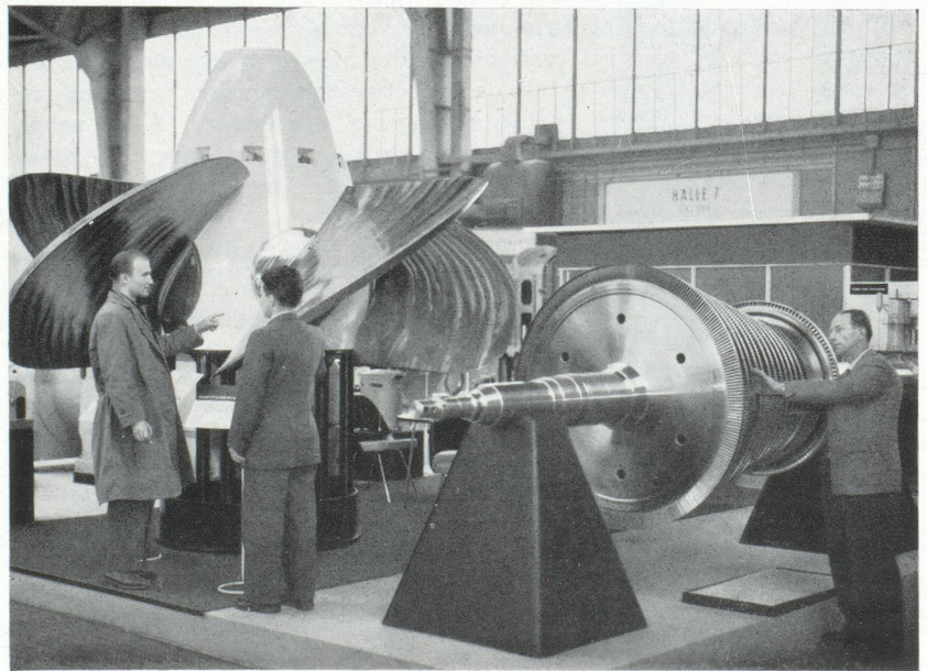
Et voici, dans le panorama offert par la grosse construction mécanique à la Foire Suisse d'Échantillons de Bâle : à gauche, une roue motrice de turbine Kaplan; à droite, un rotor pour une turbine à vapeur à haute pression. (Photo Zimmermann.)
