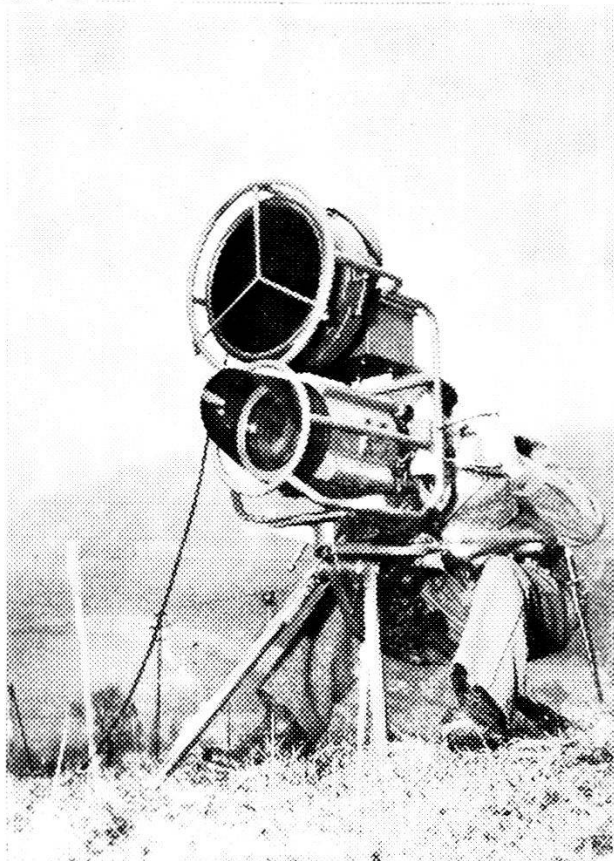
Apparecchio B 200 per osservazione a media distanza
