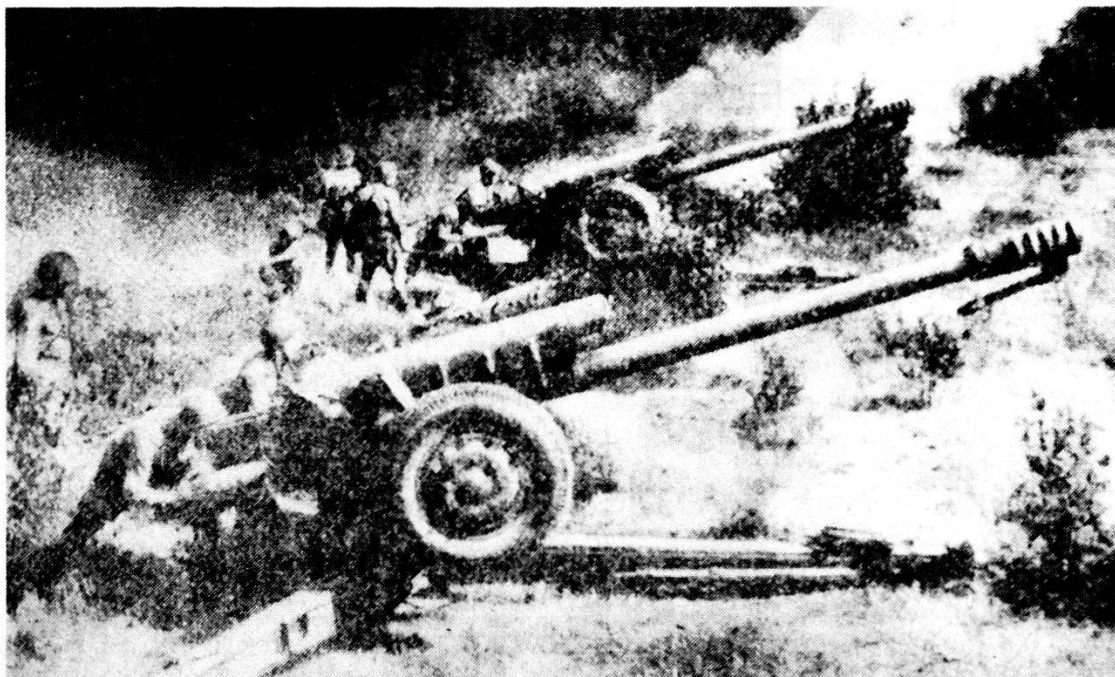
Fig. 10. L'obice M-1963 (D 30) di 122 mm. Fino a pochi anni or sono contava tra i pezzi d'artiglieria più efficienti; nelle truppe sovietiche dislocate nelle RDT viene ora sostituito con pezzi semoventi. Rimarrà in dotazione dell'esercito sovietico ancora per anni.
