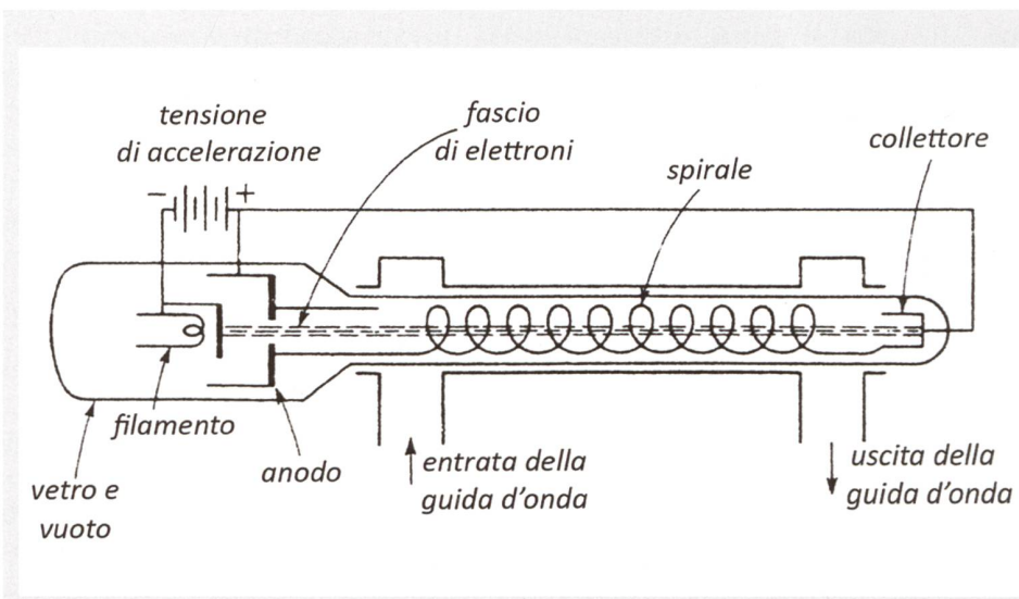
Schema della valvola TWT (©MdR).
