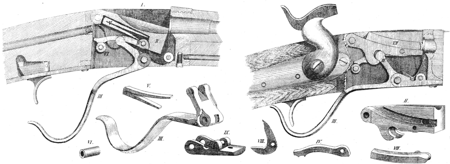
I. Boîte de Culasse. II. Obturateur. III. Pontet coudé. IV. Pièce d'arrêt. V. Ressort d'arrêt. VI. Cylindre. VII. Broche. VIII. Extracteur. IX. Support de l'Extracteur.
