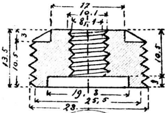
Vis - écrou.
