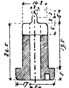
Percuteur.
