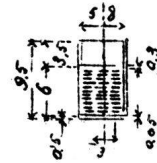
Capsule d'amorce.
