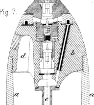
8,4 cm Shrapnel à chambre.
