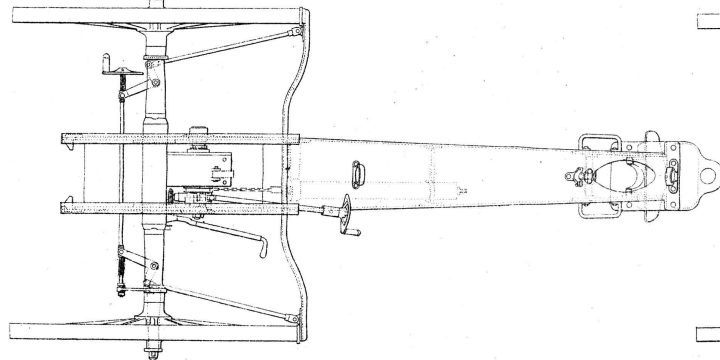
Fig. 2. Plan.
