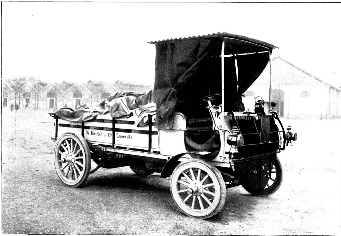
FIG. 10. — Camion de Dietrich. (Cliché de la France automobile .)
