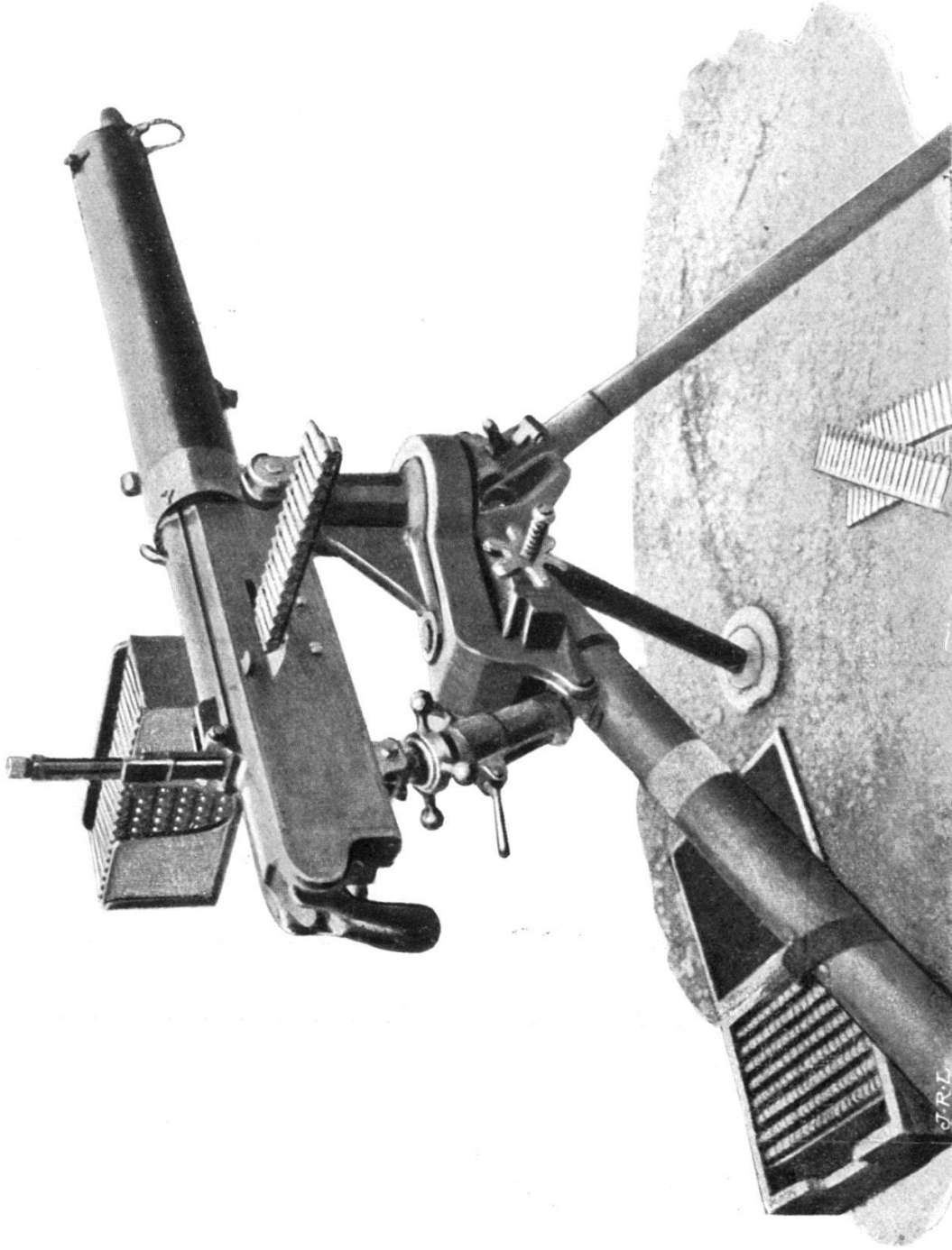
La mitrailleuse Perino.
