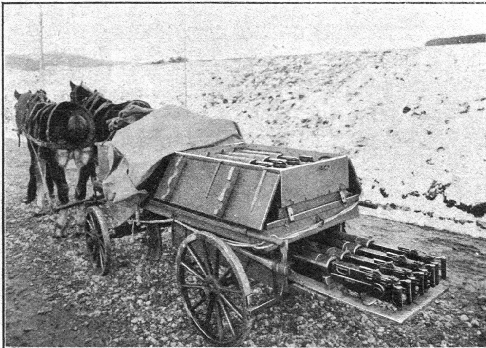
9. Gebirgsbrückenfourgon mit 8 Maschinengewehren, 8 Schildlafetten (unter der geöffneten Kiste), 32 Gurtenkisten, 8 Gewehrreffe.
