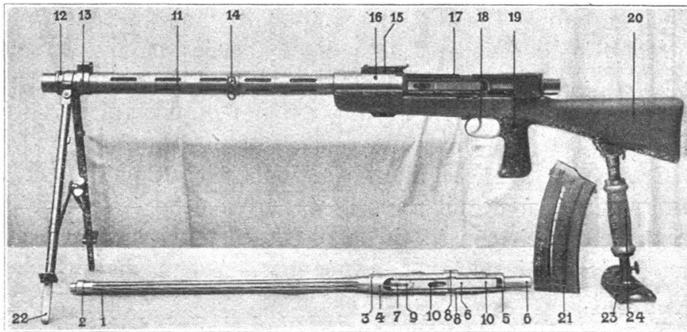
Fig. 1. Fusil Furrer monté sur deux appuis. (Côté gauche sous le fusil, canon de rechange et magasin.)
