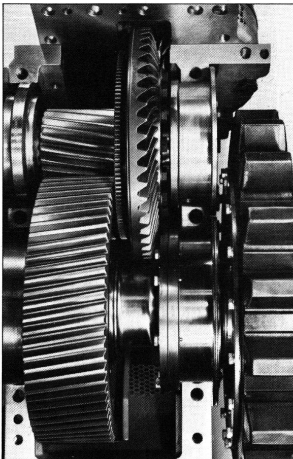
Commande de roue dentée motrice, à deux étages et avec élasticité tangentielle, pour automotrice à crémaillère pure.
