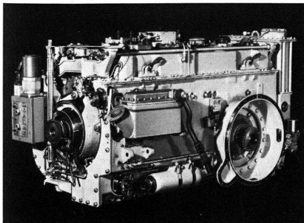
Boîte de vitesses et de direction pour véhicule lourd à chenilles, avec six vitesses en marche avant et six vitesses en marche arrière, puissance transmise 515 kW.
