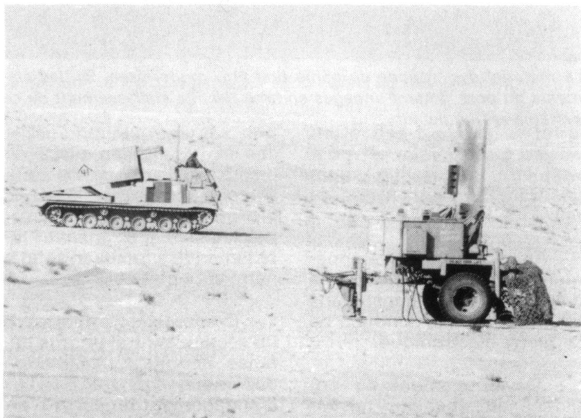
L'artillerie doit pouvoir intervenir dans la profondeur du dispositif ennemi. Il lui faut donc des moyens d'acquisition des objectifs (ici un radar de conduite du feu AN/TPQ-36 présenté à Dubaï en octobre 1991), ainsi que des missiles d'artillerie. (Photo Hughes Electronics)
