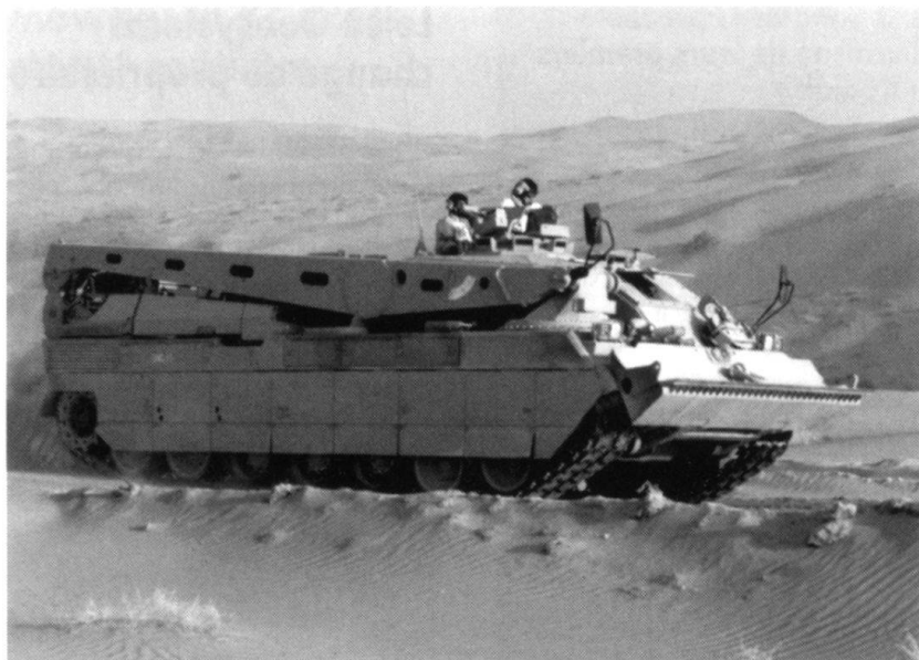
Le DNG, Dépanneur Nouvelle Génération (photo: Giat Industries)
