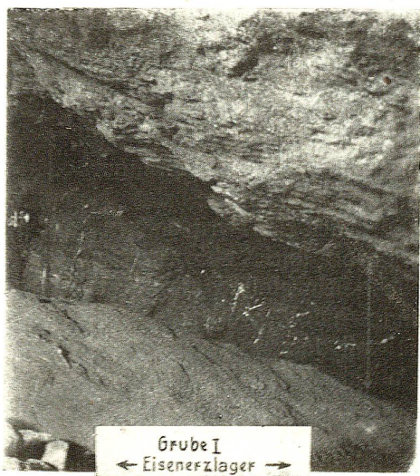
Abbildung 6. Die Erzschicht in Grube I. Ob der Erzschicht das „Hangende“, das Deckgebirge, unter der Erzschicht das Liegende.
