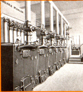
Kesselzentrale einer Hälg-Fernheizung
