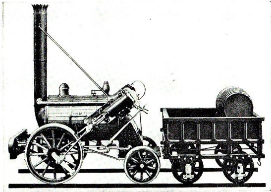
Abb. 1 Georg Stephensons Preislokomotive «Rakete», 1829; sie erreichte 55 Stundenkilometer.
