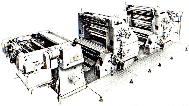
Vierfarben-Offsetpresse Roland-Ultra
