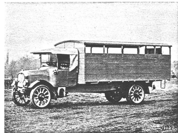
CAMION AVEC CARROSSERIE SPÉCIALE POUR LE TRANSPORT DE FROMAGE. LASTWAGEN MIT SPEZIAL-KAROSSERIE FÜR KÄSETRANSPORT. LORRY WITH SPECIAL BODY FOR THE TRANSPORT OF CHEESE.
