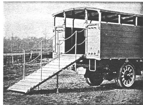
CAMION 5 TONNES POUR LE TRANSPORT DE BÉTAIL. 5 TONNEN LASTWAGEN FÜR VIEH-TRANSPORT. 5 TON LORRY FOR CATTLE TRANSPORT.
