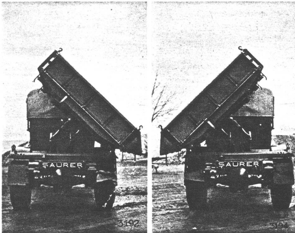
CAMION 5 TONNES AVEC BENNE BASCULANT SUR TROIS CÔTÉS. 5 TONNEN LASTWAGEN MIT DREISEITEN-KIPPBRÜCKE. 5 TON LORRY WITH 3-WAY TIPPING BODY.
