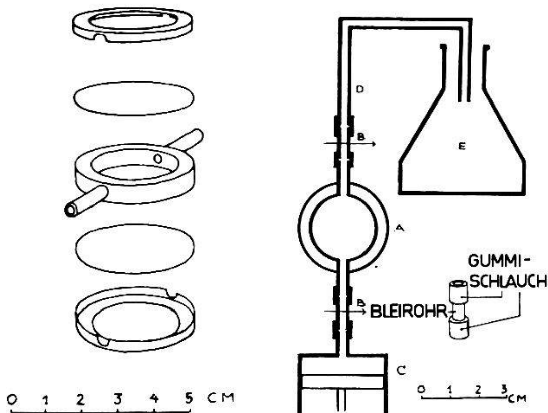
Abb. 3. Links: Cuvette zur Auszählung von \text{Kr}^{85} -haltigen Blut- und Gasproben. Stahlring mit zwei seitlichen Einfüllstutzen, oben und unten abgeschlossen durch Mica-Fenster und Halteringe. – Rechts: Füllen einer Cuvette mit \text{Kr}^{85} -haltigem Blut. A = Cuvette. C = Spritze mit \text{Kr}^{85} -haltiger Flüssigkeit. B = Gummischläuchlein, dazwischen Kupplung aus Bleiröhrchen, welche nach Füllen der Cuvetten am Ort der beiden Pfeile gequetscht werden. (Nach: Lassen N. A. und Munck O.: The cerebral blood flow in man determined by the use of radioactive krypton. Acta physiol. scand. 33, 30–49 [1955].)
