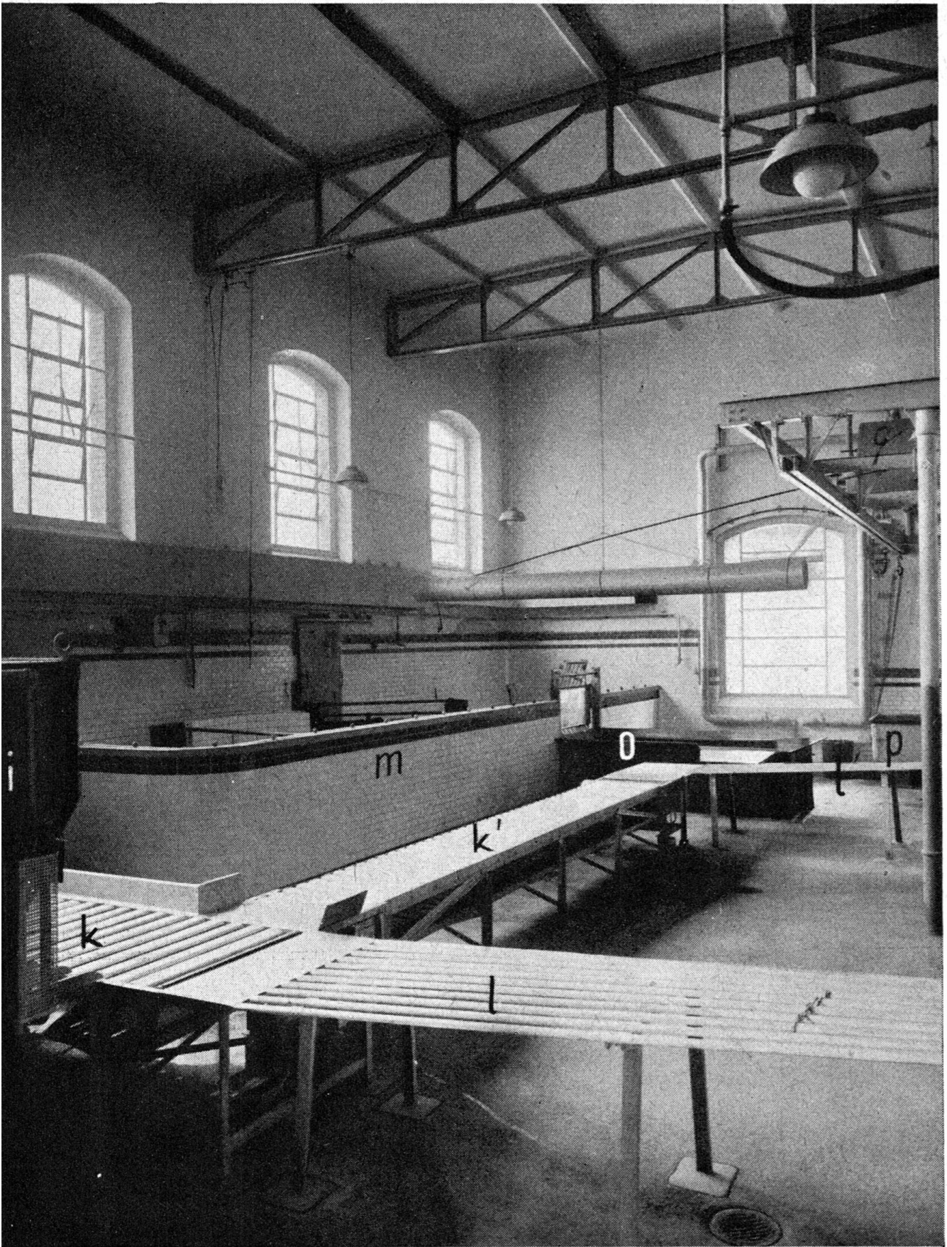
Fig. 2. Schweineschlachtanlage mit Enthaarungsmaschine (ganz links, nur teilweise sichtbar), Transport- und Enthaarungstischen. Dahinter die Reserve- und die Einzelschlachtanlage.
