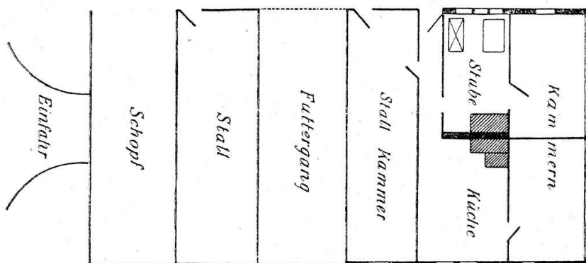
Fig. 4. (Masstab 1 : 400)
