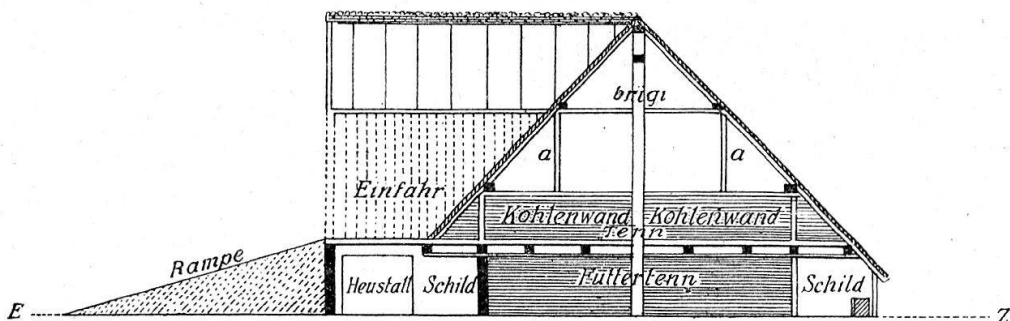
Fig. 1 g. (Masstab 1 : 350)
