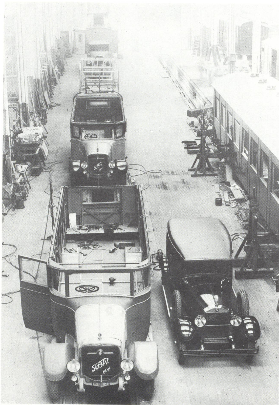
Bild 8 So sah es am 11. Juni 1929 in der Halle 3 der SIG-Waggonfabrik aus. Links eine Montagelinie von SIG-Postautomobilen mit FBW-Motoren. Vorne rechts einer der legendären MARTINI-SIX-Direktionswagen. Rechts Fertigmontage von Eisenbahnwagen für die SBB. Eine echte Diversifikation «à la carte»
