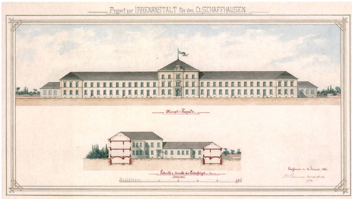
Abb. 5: Projekt für die Klinik Breitenau, Aufriss, Schnitt, Johann Christoph Bahnmaier, 26.1.1886. Aquarellierte Federzeichnung, 100×60 cm, Massstab 1 : 200. STASH SSH948-20.
