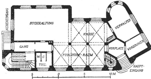
Die Ersparniskasse zu Rheinfelden. — Grundrisse vom Erdgeschoss und Wohnhof. — Maßstab 1 : 400.
