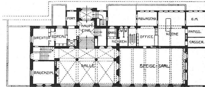
Grundrisse vom Hauptgeschoß und ersten Stof. — 1 : 500
