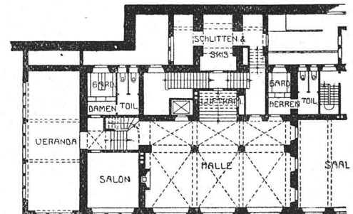
Hotel „La Margna“ in St. Moritz. — Grundrisse vom Restaurationsgeschoß und Zwischenstof. — Maßstab 1 : 500
