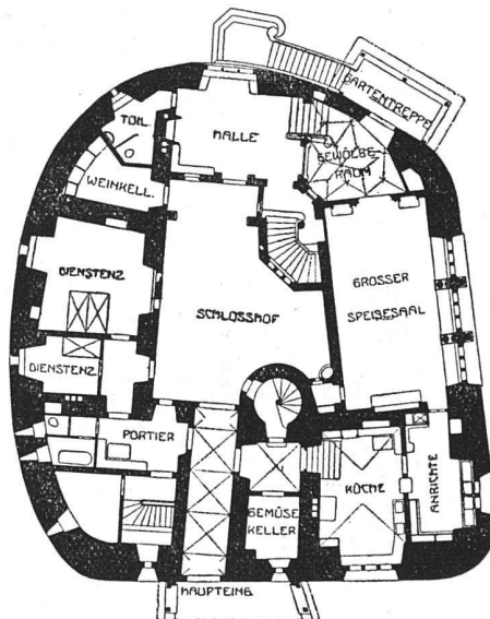
Grundriß vom Erdgeschoß
