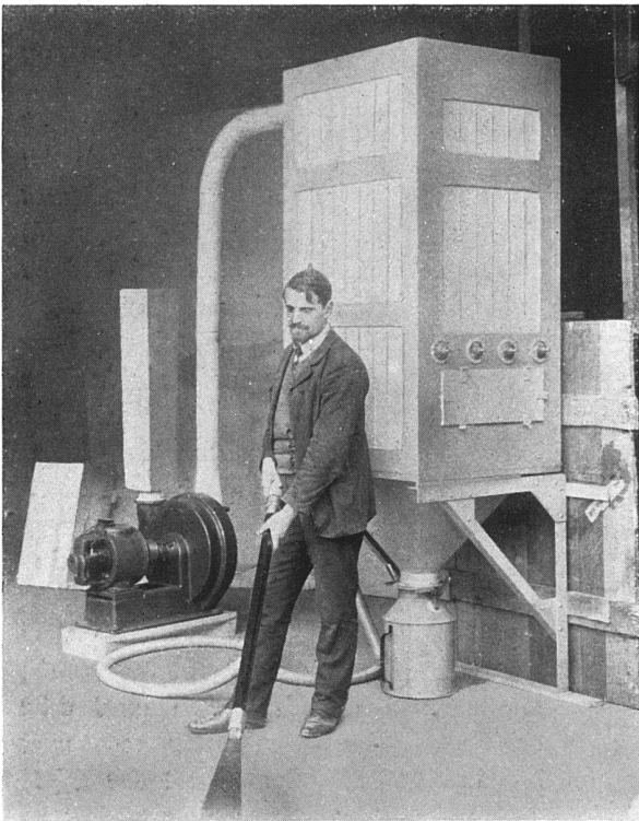
Abb. 17. Stationäre pneumatische Reinigungsanlage mit Zweistufenturbine und Filterkasten mit Ablappvorrichtung von Meidinger & Co., Basel. (Vergl. Zeichnung und Text S. 226)
