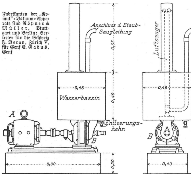
Fabrikanten der „Romul“-Vakuum-Apparate sind R ö p n e r & M ü l l e r, Stuttgart und Berlin; Vertreter für die Schweiz F. B e r a n, Zürich V. für Genf E. G a b u s, Genf D. R.-Patent Abb. 21. „Romul“-Vakuum-Apparat, durch Elektromotor betrieben. — Maßstab 1 : 20 Schweizer-Patent
