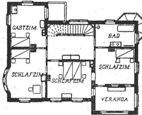
Grundrisse. — Maßstab 1:400.
