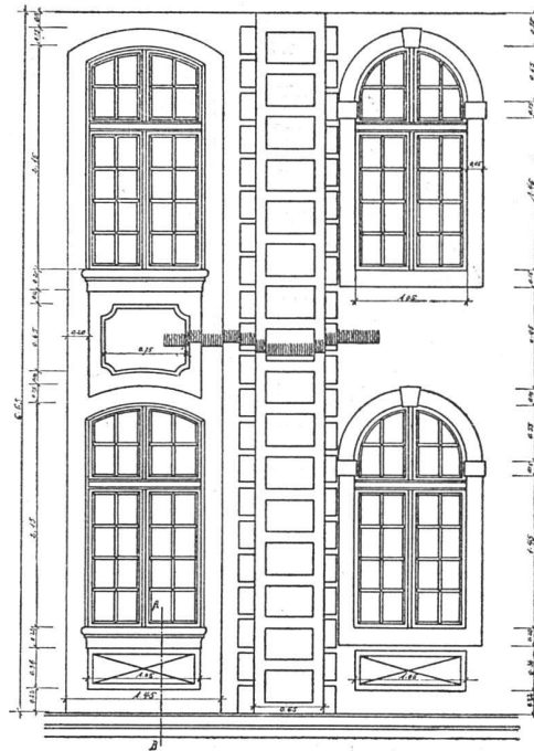
Detail der Hauptfassade 1:75
