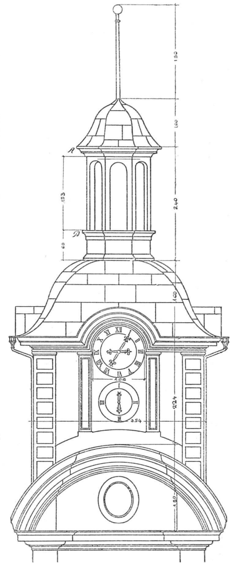
Aufriß und Schnitt des Turmes. — Maßstab 1:75
