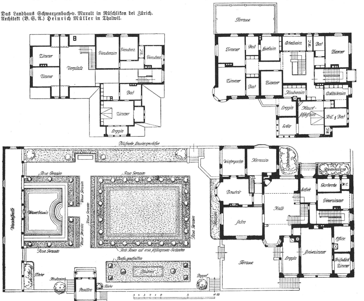
Grundrisse vom Keller, Erdgeschoss, ersten Stock und Dachboden. Maßstab 1:400. — Der Hausgarten ist von dem Gartenbau- geschäft Otto Fröbels Erben in Zürich V angelegt worden.
